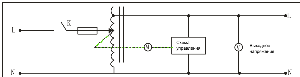
Рисунок 2: Принципиальная схема модели CH-93010.
