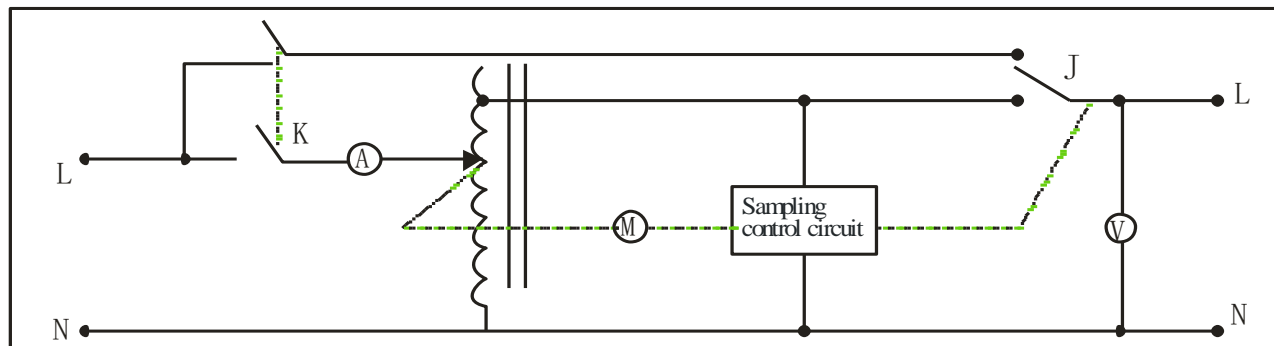
Рисунок 3: Принципиальная схема модели CH-93020 и CH-93030.
