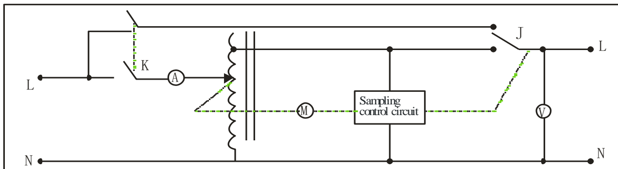
Рисунок 3: Принципиальная схема модели PS9302 и PS9303.
