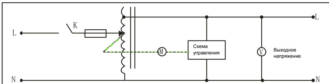
Рисунок 2: Принципиальная схема модели PS9301.
